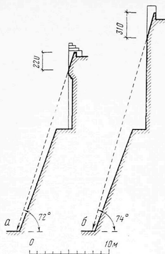
Рис. 17. Определение уклонов бойниц и их размеров по фасаду
