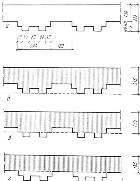
Рис. 11. Внешняя стена Центрального массива дворца в месте примыкания Южного массива
