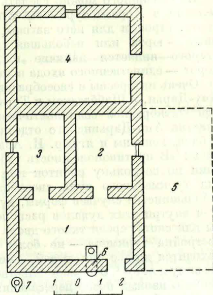
Рис. 5. План жилого дома (Калининский р-н Ташаузской обл.).
