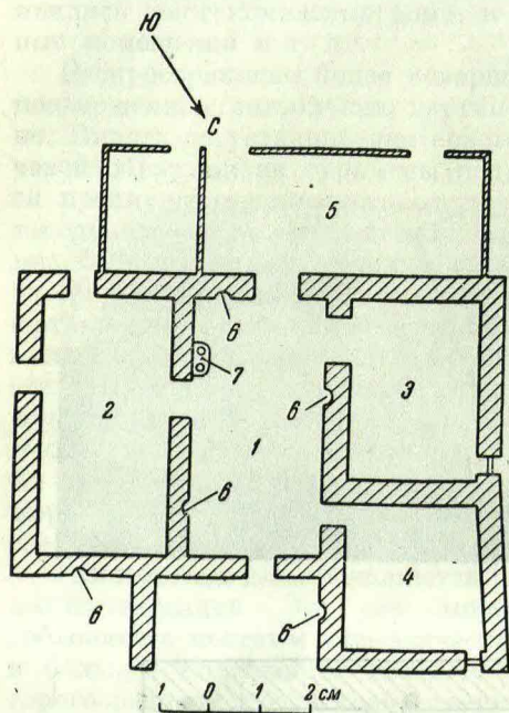
Рис. 2. План жилого дома (Дарган-Атинский р-н, аул Садыбар).
