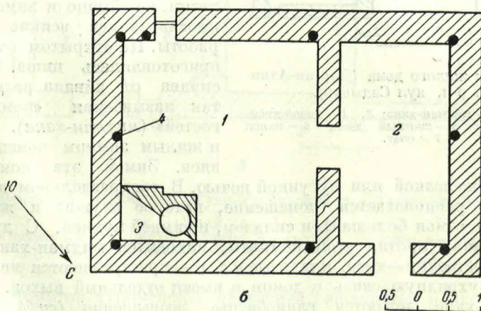
Рис. 1. «Там-кепше» — постройка старого типа (Дарган-Атинский р-н Чарджоуской обл. ТССР): а — общий вид; б — план.
