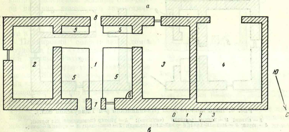
Рис. 3. Современный жилой дом (Куны-Ургенчский р-н Ташаузской обл. ТССР)
