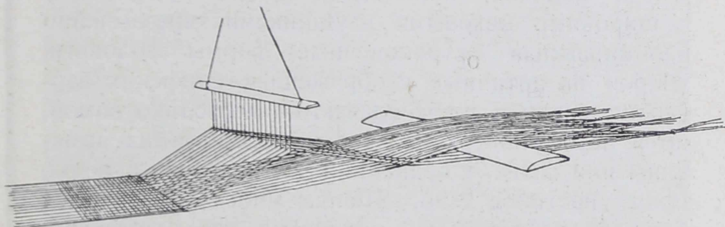
Схематический чертеж положения нитей при тканье. (Положение первое).
