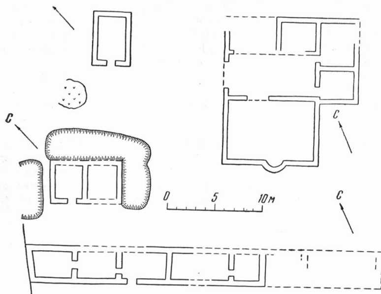
Рис. 5. Крепость Машрык-Сенгир. Типы жилых домов.
