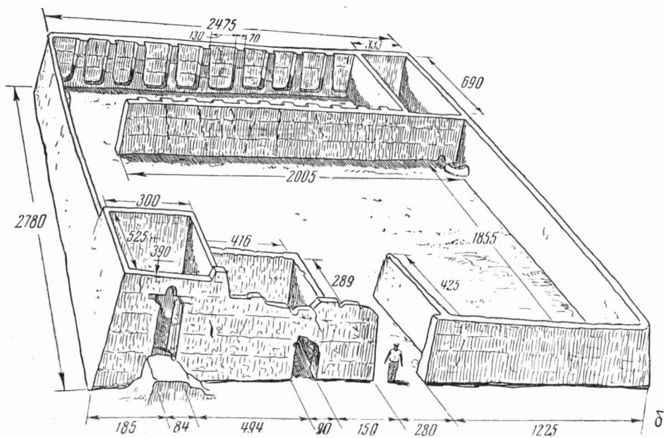
Рис. 3. Усадьба туркмена коджука (урочище Уаз): а — внешний вид; б — перспективный план.
