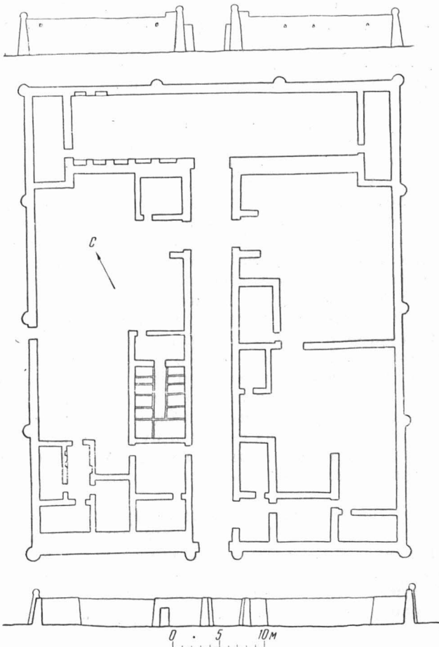
Рис. 2. Усадьба туркмена-емрели (урочище Уз): a — главный вход; b — план усадьбы.
