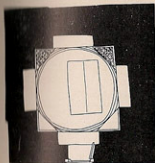
Мавзолей хорезмшаха Иль-Арслана (Фахр-ад-дин Рази). Планы по четверику и восьмигранному барабану. По обмеру Н. Бакланова, 1929 г. АксонOMETрический разрез. По чертежу Н. Бакланова, 1929 г.
