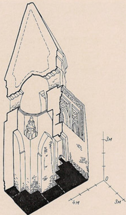
Мавзолей хорезмшаха Иль-Арслана (Фахр-ад-дин Рази). Планы по четверику и восьмигранному барабану. По обмеру Н. Бакланова, 1929 г. АксонOMETрический разрез. По чертежу Н. Бакланова, 1929 г.
