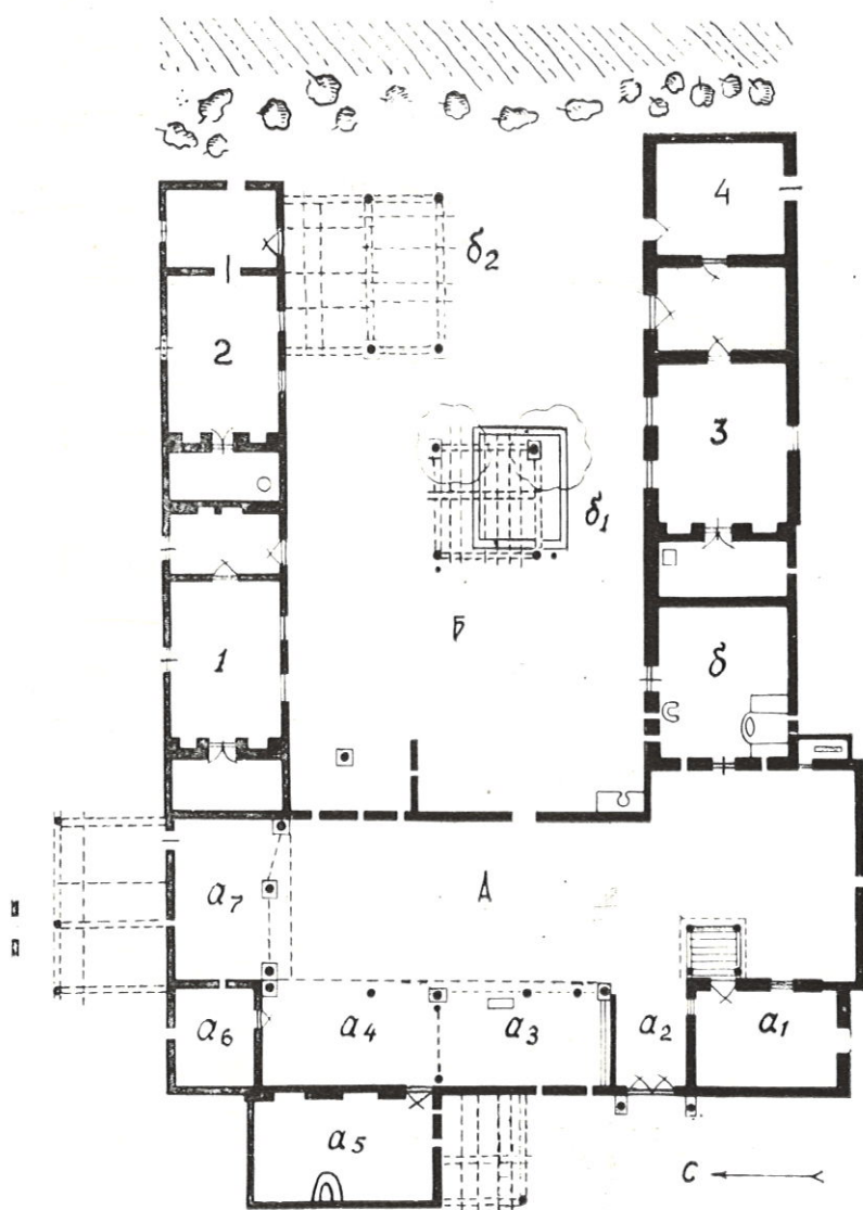
Рис. 1. План усадьбы (кишлак Убо, Урмитганский р-н). 1, 2, 3 — жилые трехкамерные помещения; А — хозяйственная часть усадьбы (берун); a_1 — мехмонхона; a_2 — дарвозахона; a_3 — айвон; a_4 — айвон; a_5 — оғил; a_6 — айвон; a_7 — айвон; Б — жилая часть усадьбы (дарун); б — ошхона; \delta_1 — гулзор; \delta_2 — толор.
