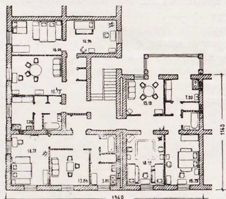
Угловая секция 3-2-3 Жилая площадь 132,94 м 2 Полезная площадь 200,98 м 2 Строительный объем 1021,8 м 3
