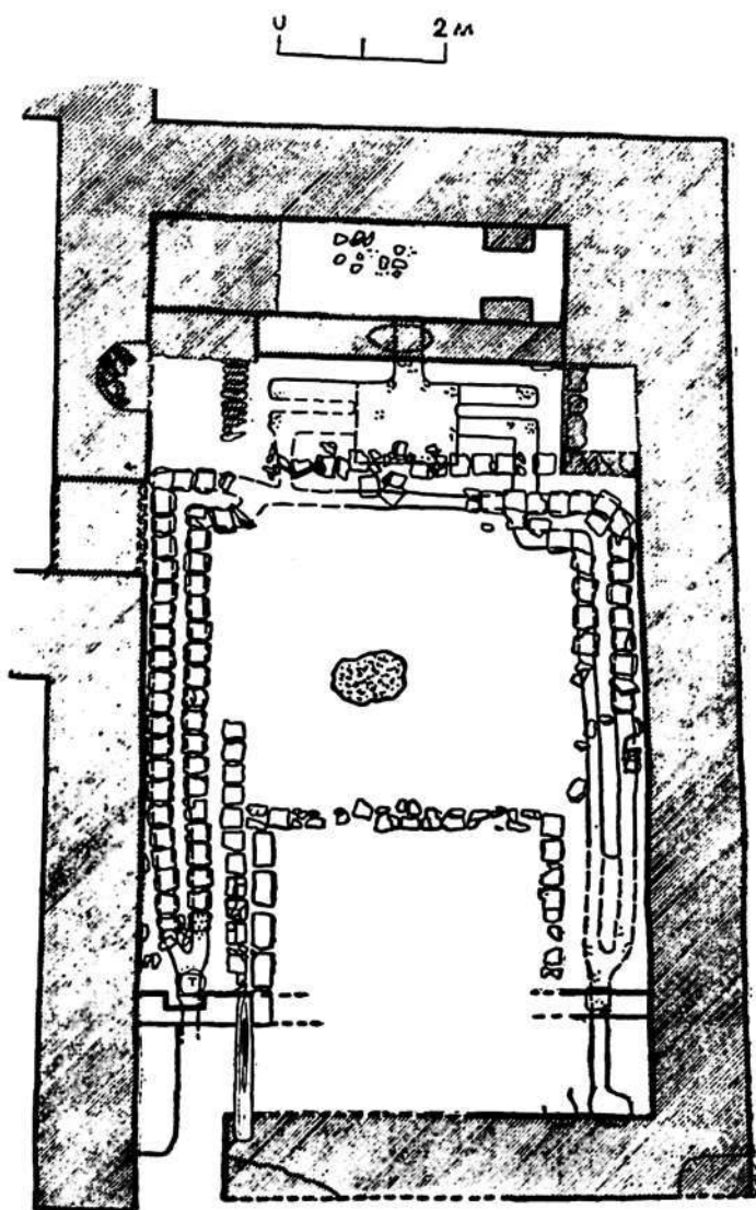
Рис. 4. Отопительная система в помещении 5.
