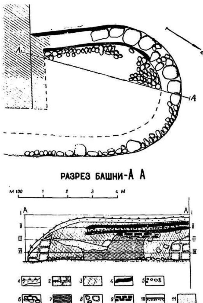
Рис. 4. План и разрез угловой башни.
