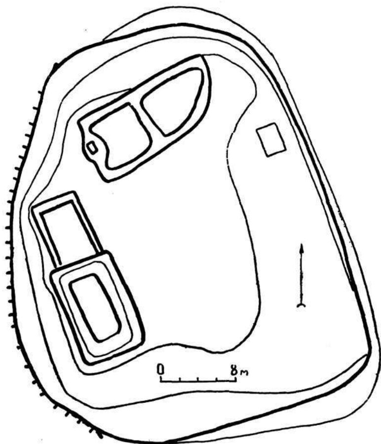
Рис. 7. План городища Кум-Арык.
