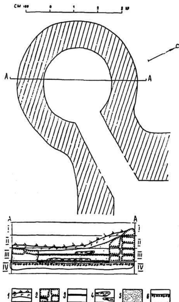
Рис. 5. План и разрез угловой башни цитадели.
