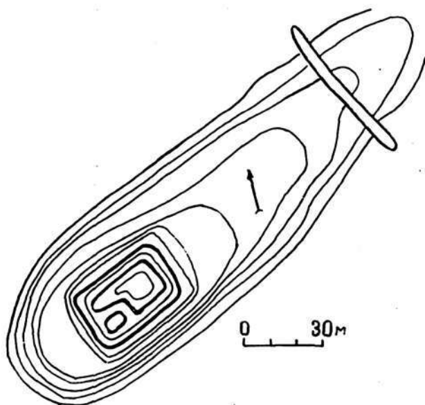
Рис. 13. План городища Котур-Сай I.
