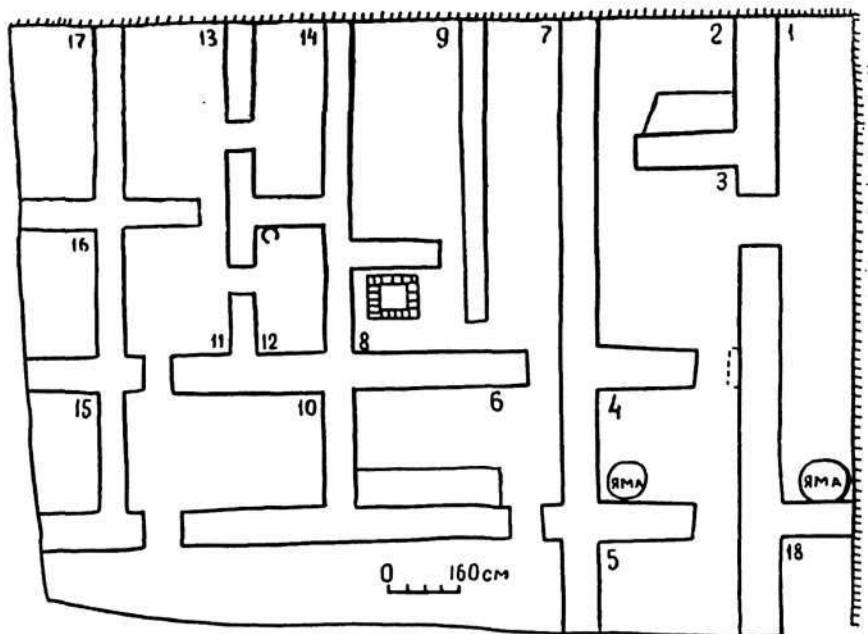
Рис. 2. План второго строительного горизонта.
