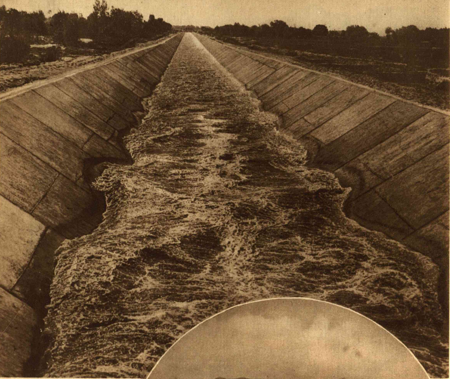
Главный водосток плотины имени 1-го мая Фото А. Шайхета
