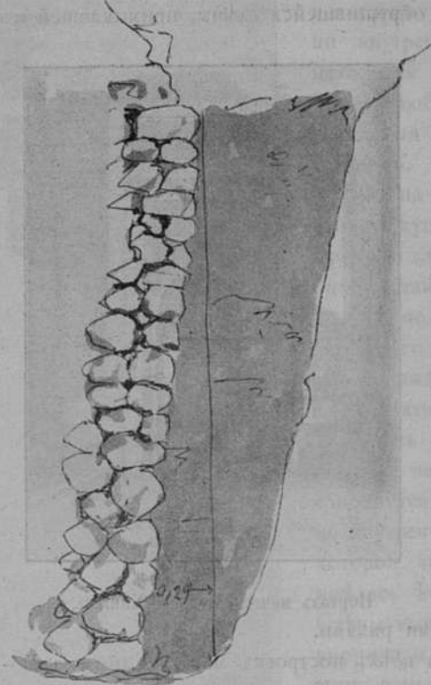
Фундаментъ минарета.
