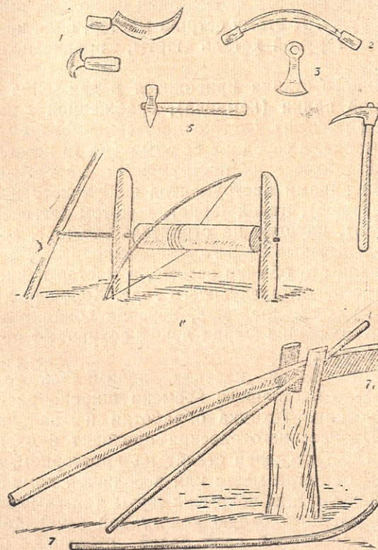
Рис. 12. Инструменты для выделки остова юрт. 1—сапожные ножи (кесер); 2—рубанок (ренде); 3—тесло (теше); 4—тесло с деревянной ручкой (теше); 5—молоток (чекич); 6—станок для сверления (перми); 7—приспособление для сгибания жердей (дукан); 7а—рабочая часть рычага дукана (хачча).
