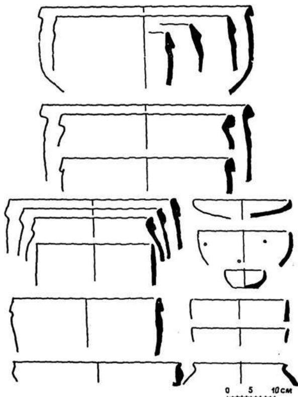
Рис. 5. Керамический комплекс периода Кучук—IV.
