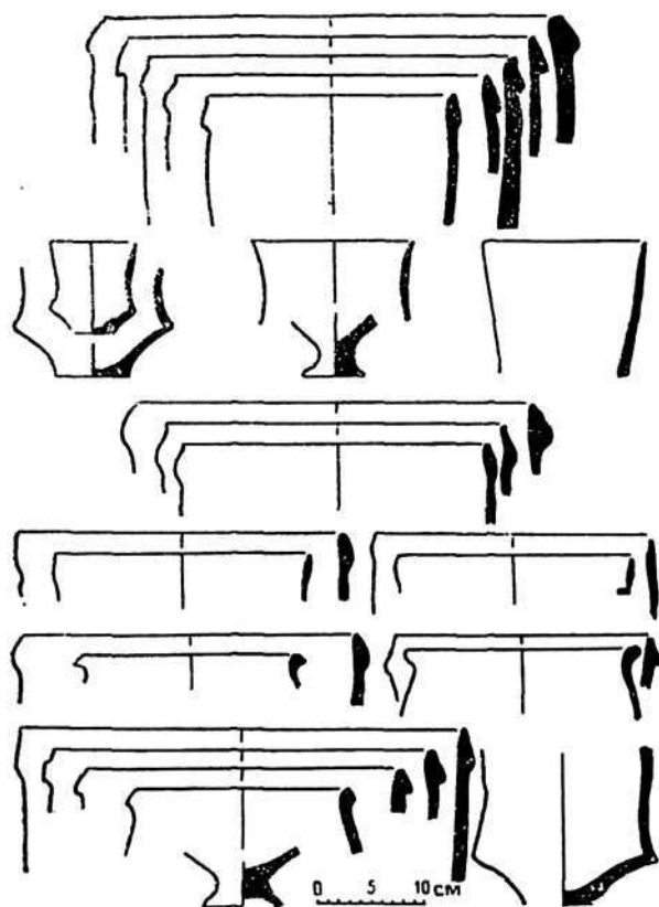
Рис. 4. Керамический комплекс периода Кучук—III.
