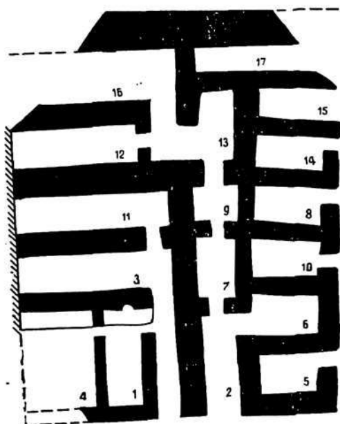
Рис. 1. План замка.
