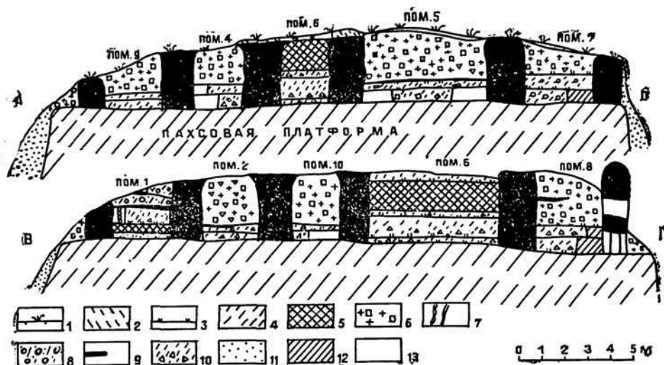
Рис. 2. Разрезы:
