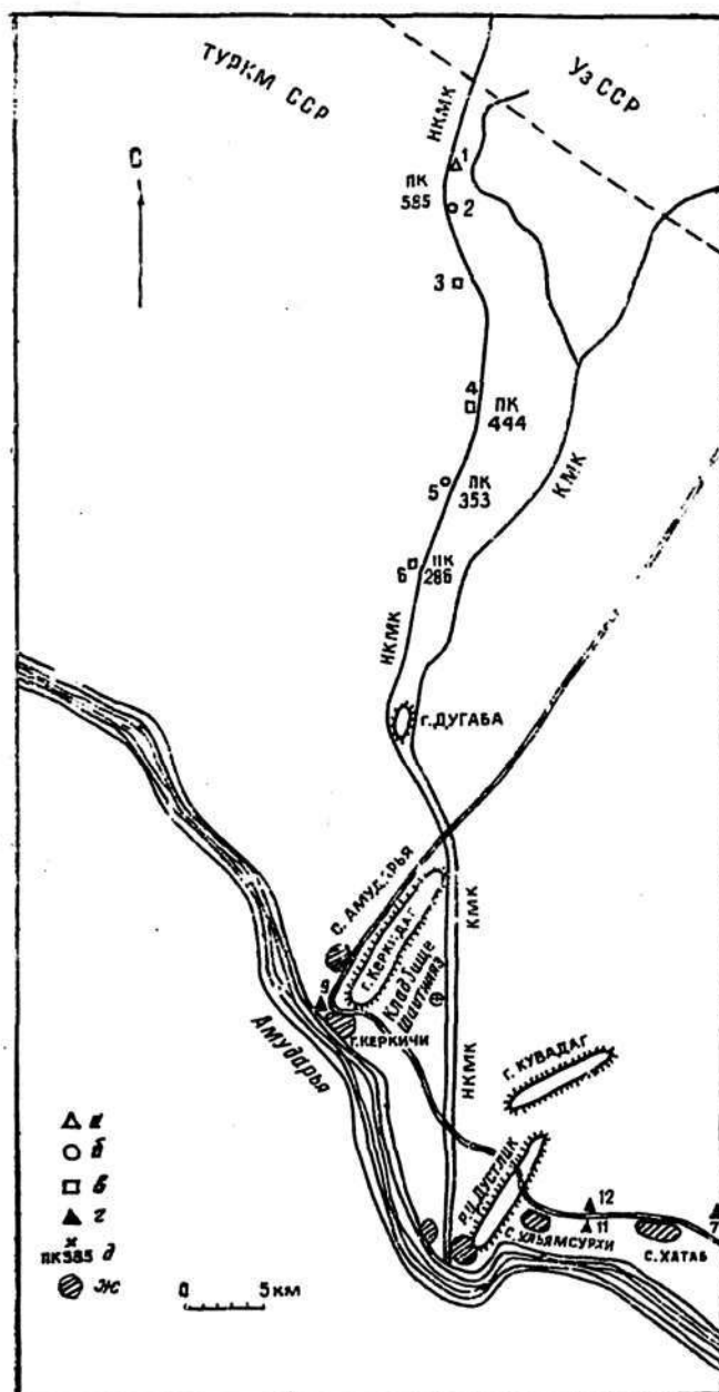
Рис. 1. План трассы НКМК от границ УзССР до Амударьи:
