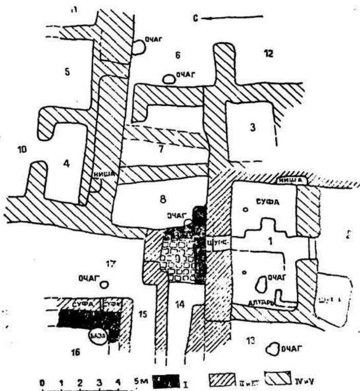
Рис. 1. План жилого комплекса.
