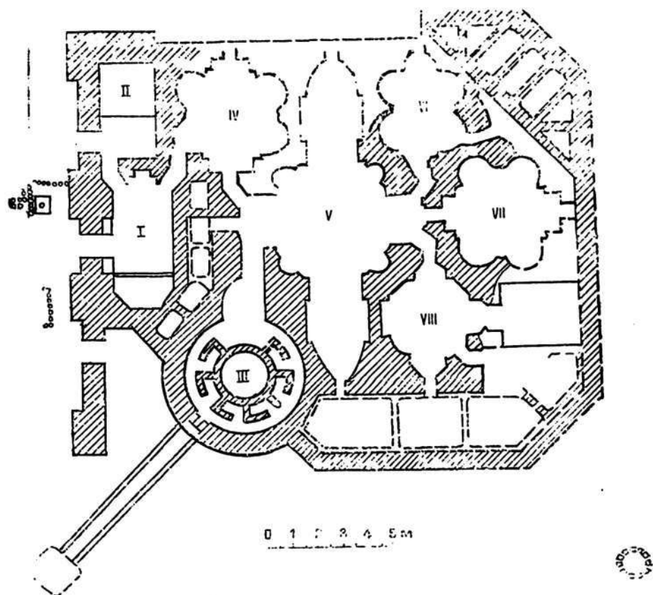
Рис. 2. Реконструкция планировки бани.
