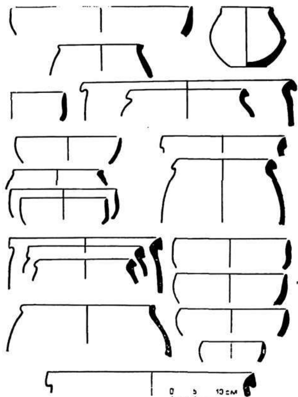
Рис. 3. Керамический комплекс периодов Кучук—I 6, II.
