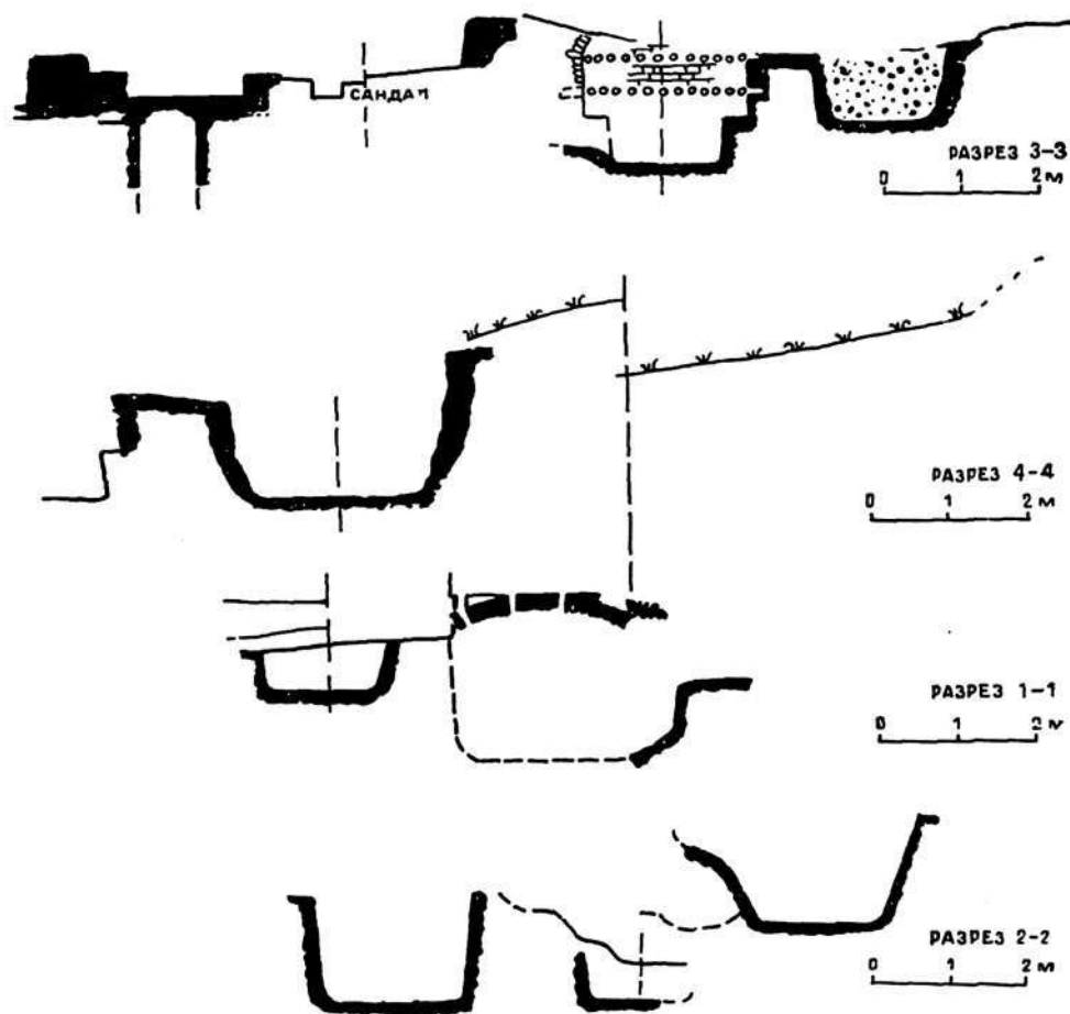
Рис. 2. Мастерские керамистов. Разрез.
