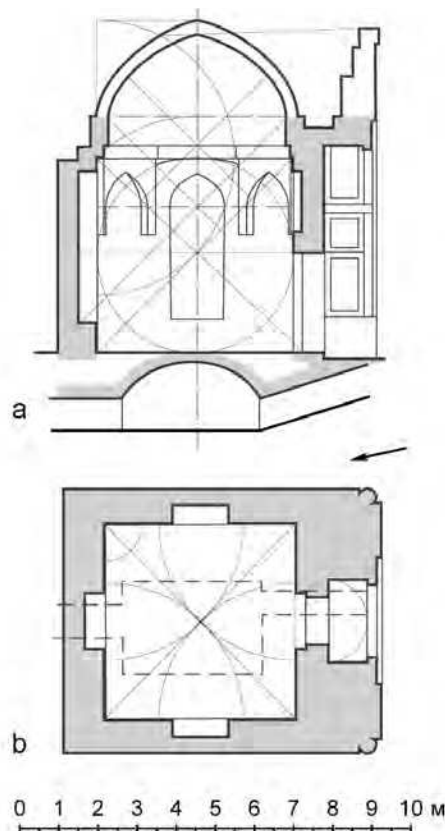
Рис. 105. Мавзолей Ходжи Ахмада: а – разрез, b – план (по Ю.З. Шваб)
