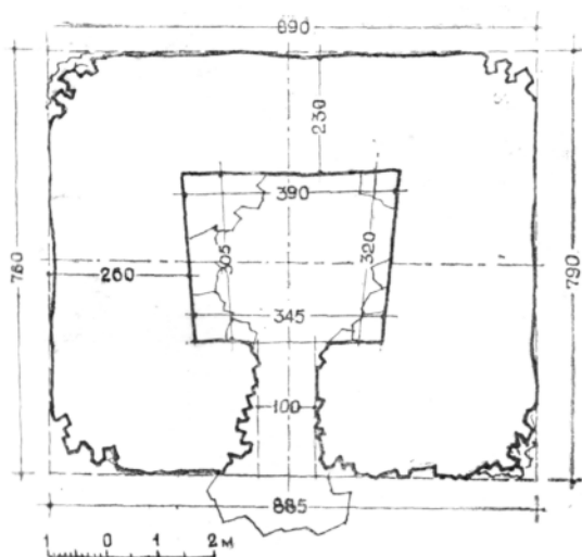
Рис. 2 .Мавзолей Домбаул. План.
