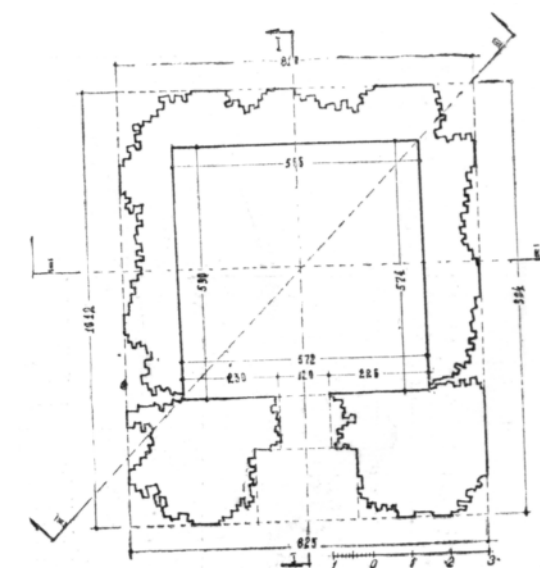
Рис. 9. Мавзолей Аяк-Хамыр. План на отметке \sim 0,00 .
