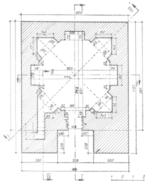
Рис. 23. Мавзолей Алаша-хан.. План на отметке \pm 0,00 .
