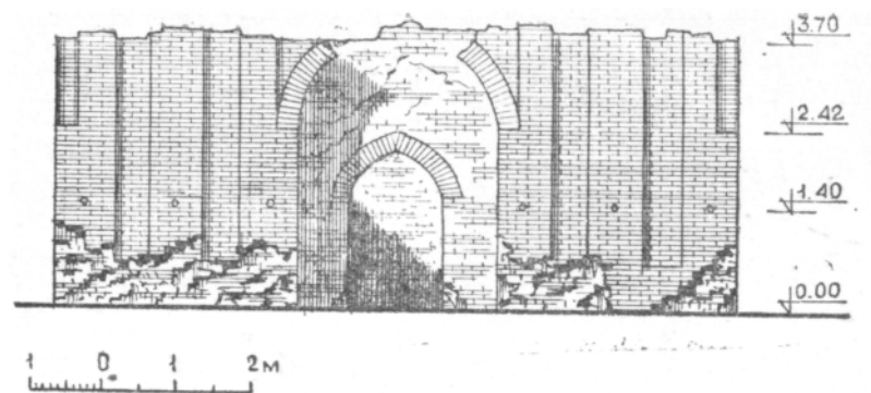
Рис. 40. Мавзолей Болган-ана. Главный фасад.
