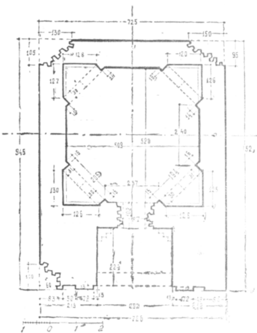
Рис. 34. Мавзолей Джоши-хан. План на отметке + 1,10.
