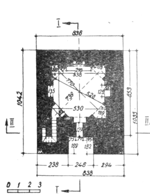
Рис. 49. Мавзолей Жузень План.
