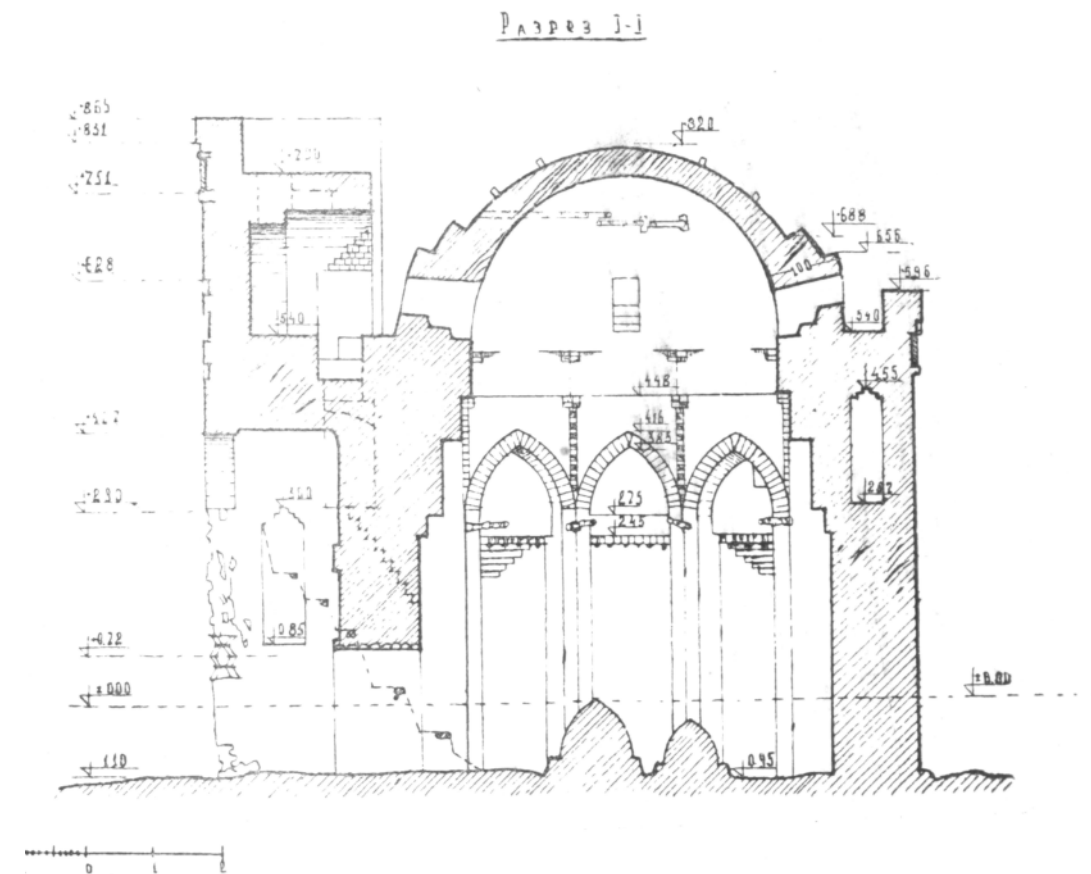
Рис. 57. Мавзолей Жузденъ. Продольный разрез.
