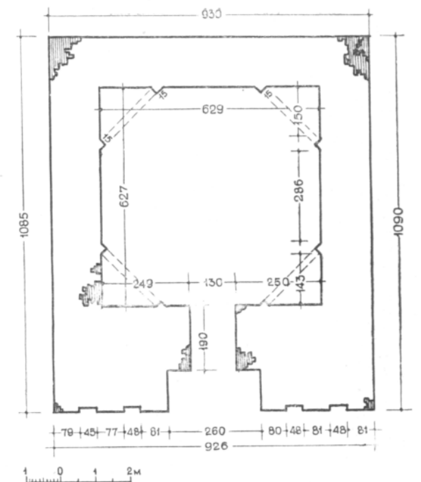
Рис. 39. Мавзолей Болган-ана. План.
