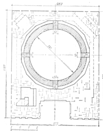
Рис. 26. Мавзолей Алаша хан. План купола.
