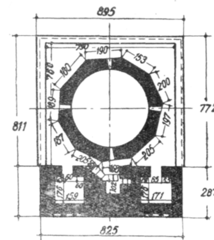
Рис. 51. Мавзолей Жузень. План подкупольного барабана.
