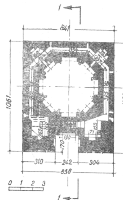
Рис. 50. Мавзолей Жузень, План второго этажа. Галерея.
