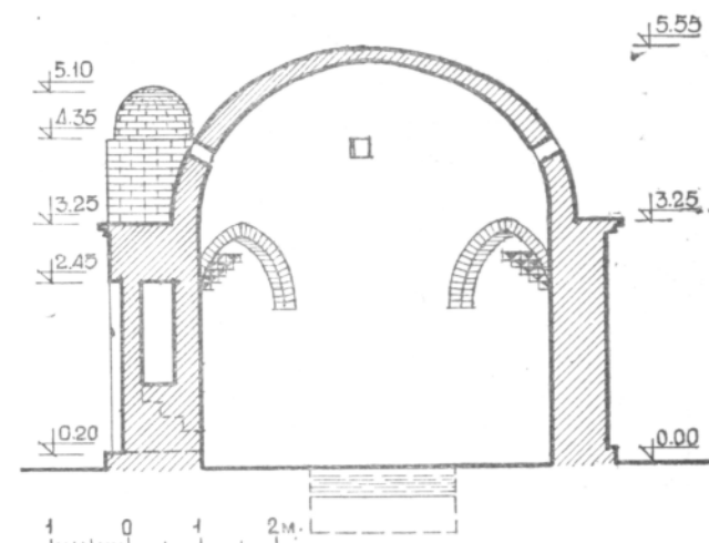
Рис. 74. Мавзолей Дюсембек. Разрез.
