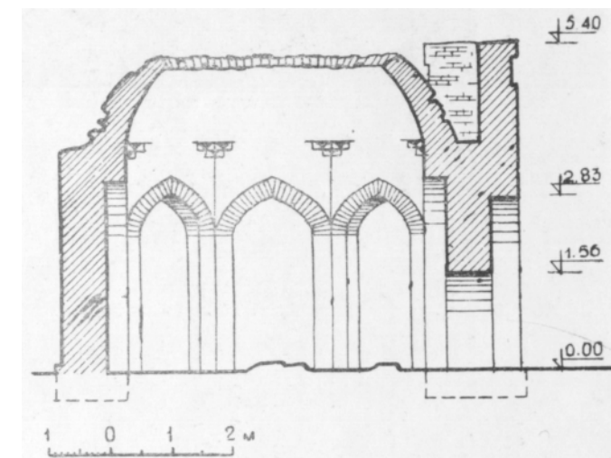
Рис. 44. Мавзолей Тулек. Разрез.
