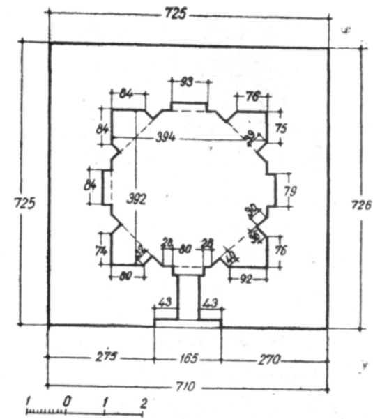
Рис. 63. Мавзолей Торг-Кара. План.
