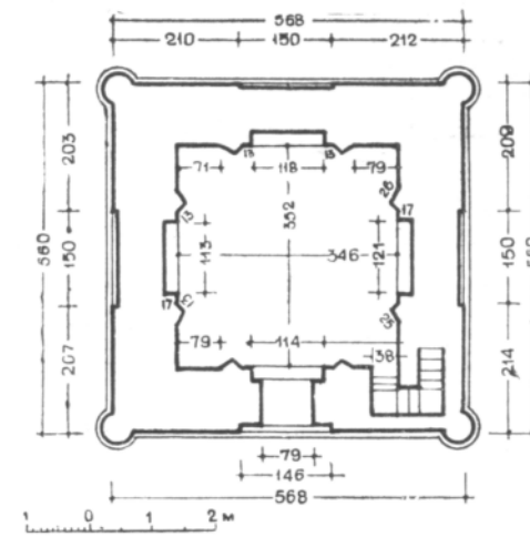
Рис. 89. Мавзолей Жерапай-Майкин. План.
