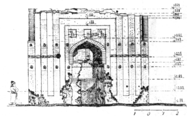
Рис. 7 .Мавзолей Аяк-Хамыр. Главный фасад.
