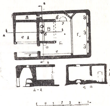
Рис. 37. План и разрез дома Рахматуллоева X., к. Маргиб:
