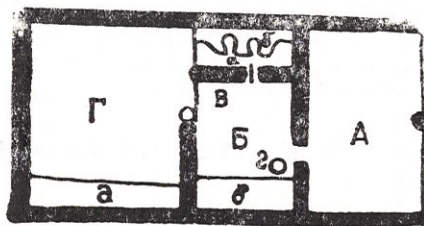
Рис. 48. План дома Икрамова Накиба, к. Вору: А — айвон ; Б — прихожая — кавшпарт ; В — очажное отделение — мур ; Г — чистое отделение — рухона ; а — очаг для приготовления пищи — сангупоча ; б — очаг-печь для печения лепешек — оштон ; в — глинобитное возвышение для дров — суфай хезумгирий ; г — яма-поглотитель — обрез ; д — возвышение для постельных принадлежностей — суфай курпатахкун .
