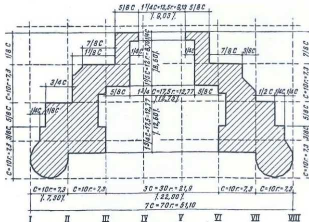
Рис. 84. Шахриябз. Анализ построения плана портала дворца Ак-Сарай.
