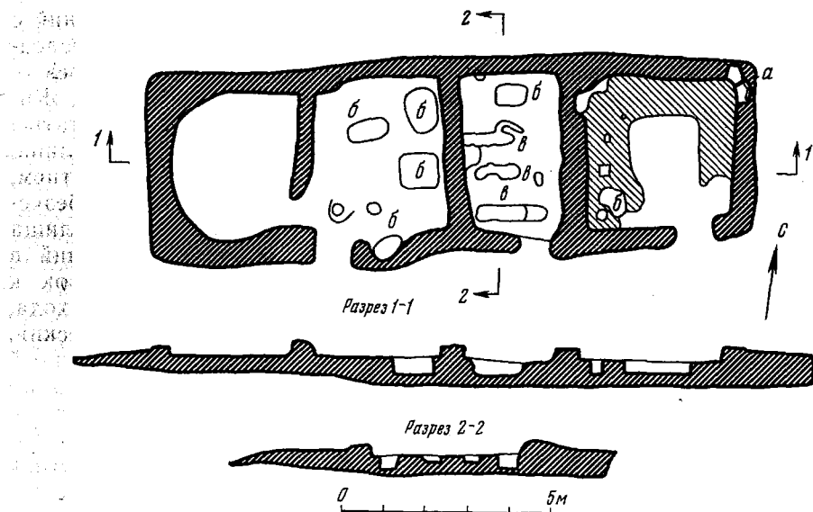
Рис. 5. Дом в поселении XIV в. близ Дэв-калы
