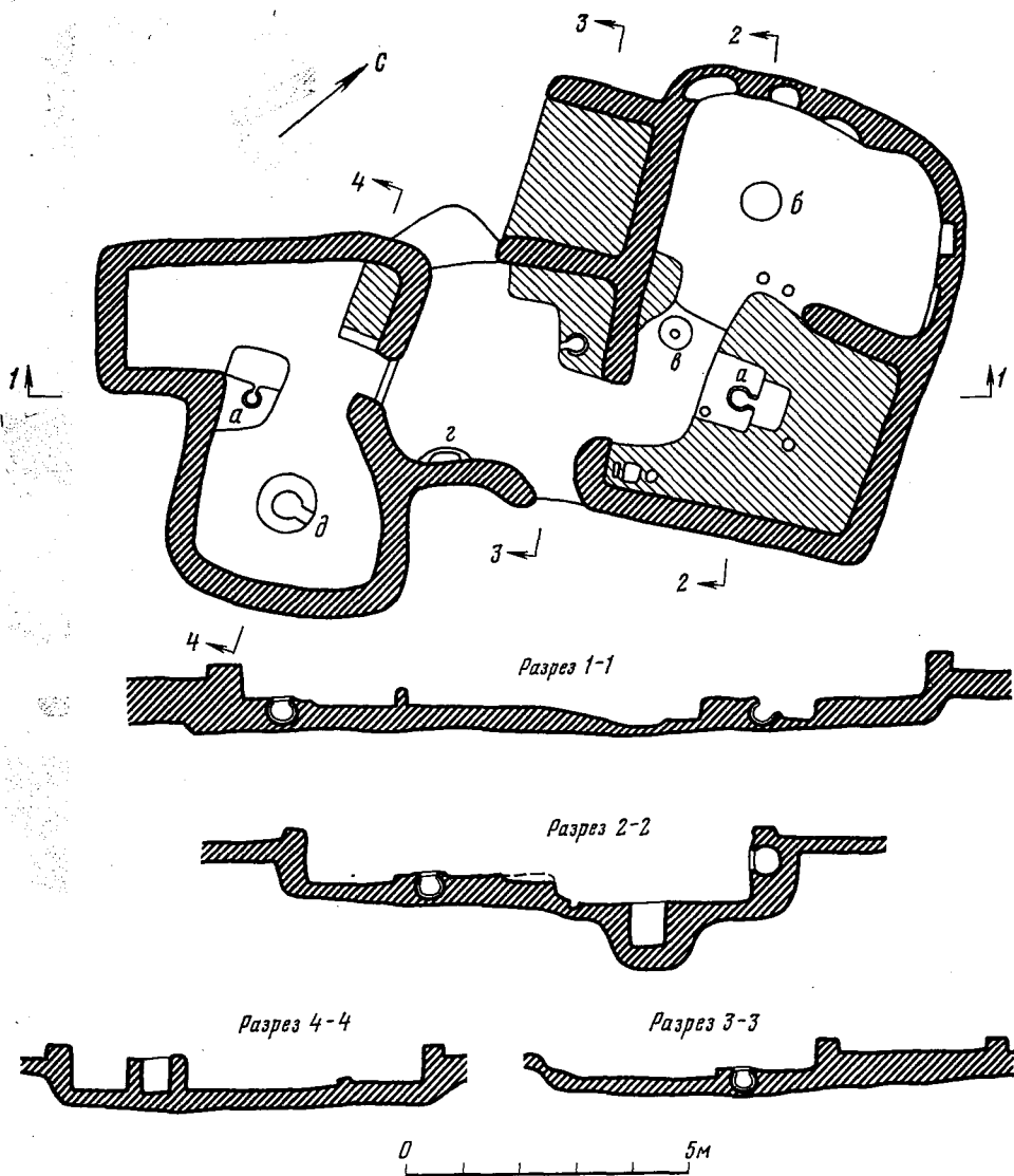
Рис. 4. Дом № 2 в Куня-Узском поселении середины XIV в.
