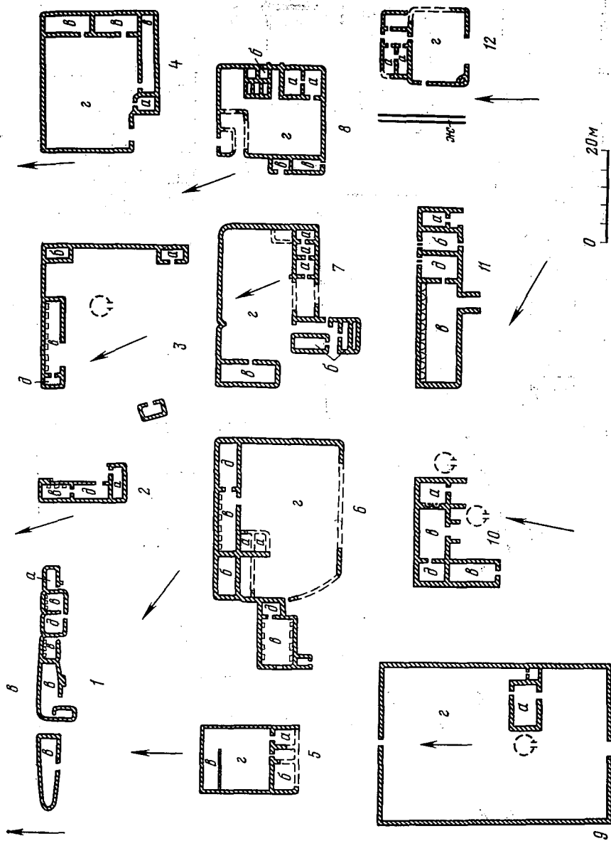
Рис. 1. Типы туркменских усадеб 1, 2 — урочище Ат-Крылган. Усадьбыг вблиз селгиря (укрепления) туркмен-орсуки; 3, 6, 10, 12 — усадьбы вблиз Катакар-Чардере; 4, 9 — урочище Ат-Крылган; 5 — усадьба в районе Саккар-яба; 7, 8 — усадьбы в районе Чатыр-яба (салаки?); 11 — урочище Ат-Крылган. Усадьба Чалмергена окуз); а — жилые помещения, б — кладовые (телеки, учеки), в — помещения для скота (ат-хана, сенс-хана и др.), г — дворы, д — помещения для сена (саман-хана), е — водоемы (хаусы), ж — ары-ки, и — помещение мечети. Площадки для юрт, различные на местности, отмечены пунктиром
