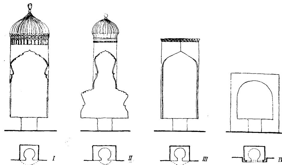
Рис. 82. Камини ферганских домов
