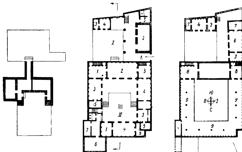
План подвала
