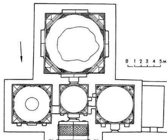
3. Куля-Ургенч. Мавзолей Наджмеддин Кубра. Северный фасад, разрез север—юг, план
