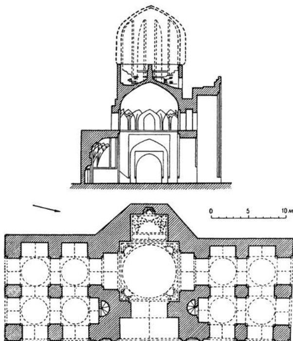
15. Карши. Мечеть-намазга, XVI в. Разрез, план
