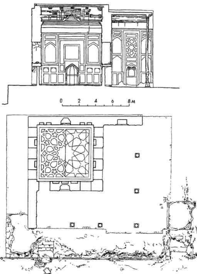
5. Бухара. Мечеть Баянд, XVI в. Общий вид, разрез, план
