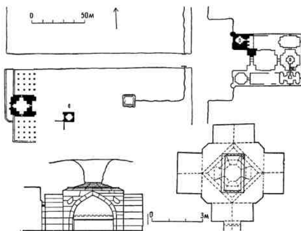
7. Шахрисябз. Ансамбль Доруссиадат, конец XIV в. Пилон входного портала с мавзолеем Джехангира, интерьер мавзолея Джехангира, план ансамбля, разрез и план склепа
