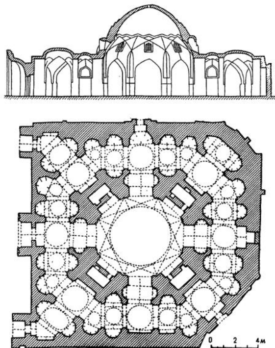
14. Бухара. Тим Абдулла-хана, XVI в. Разрез, план
