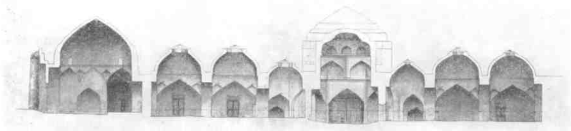
14. Хива. Рынок Алла-Кули-хана. Разрез
