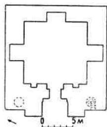
16. Меана (Туркменистан). Мавзолей Абу-Саида, XI в. Общий вид, разрез, план
