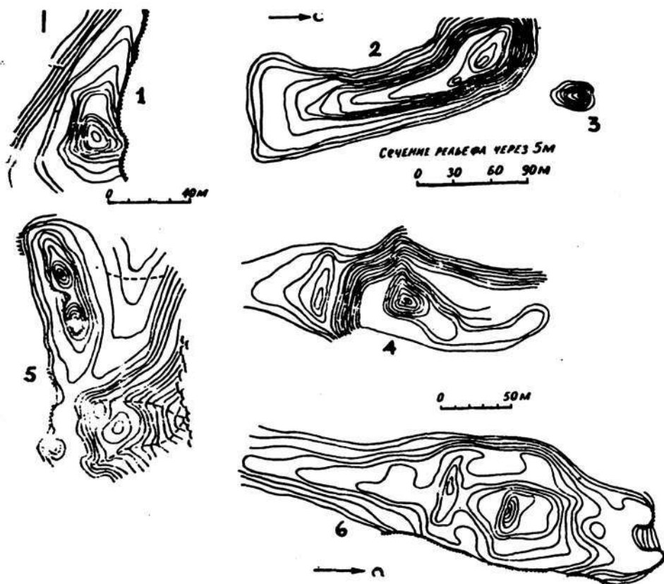
Рис. 9а. Топографические планы: 1—Калаан Хосров; 2—Калаан Муг (в к. Амондара по О. И. Смирновой); 3—Тепан Муг; 4—Калаан Рустам; 5—Калаан Муг в к. Шашкот; 6—Калаан Мир в к. Кулоли
