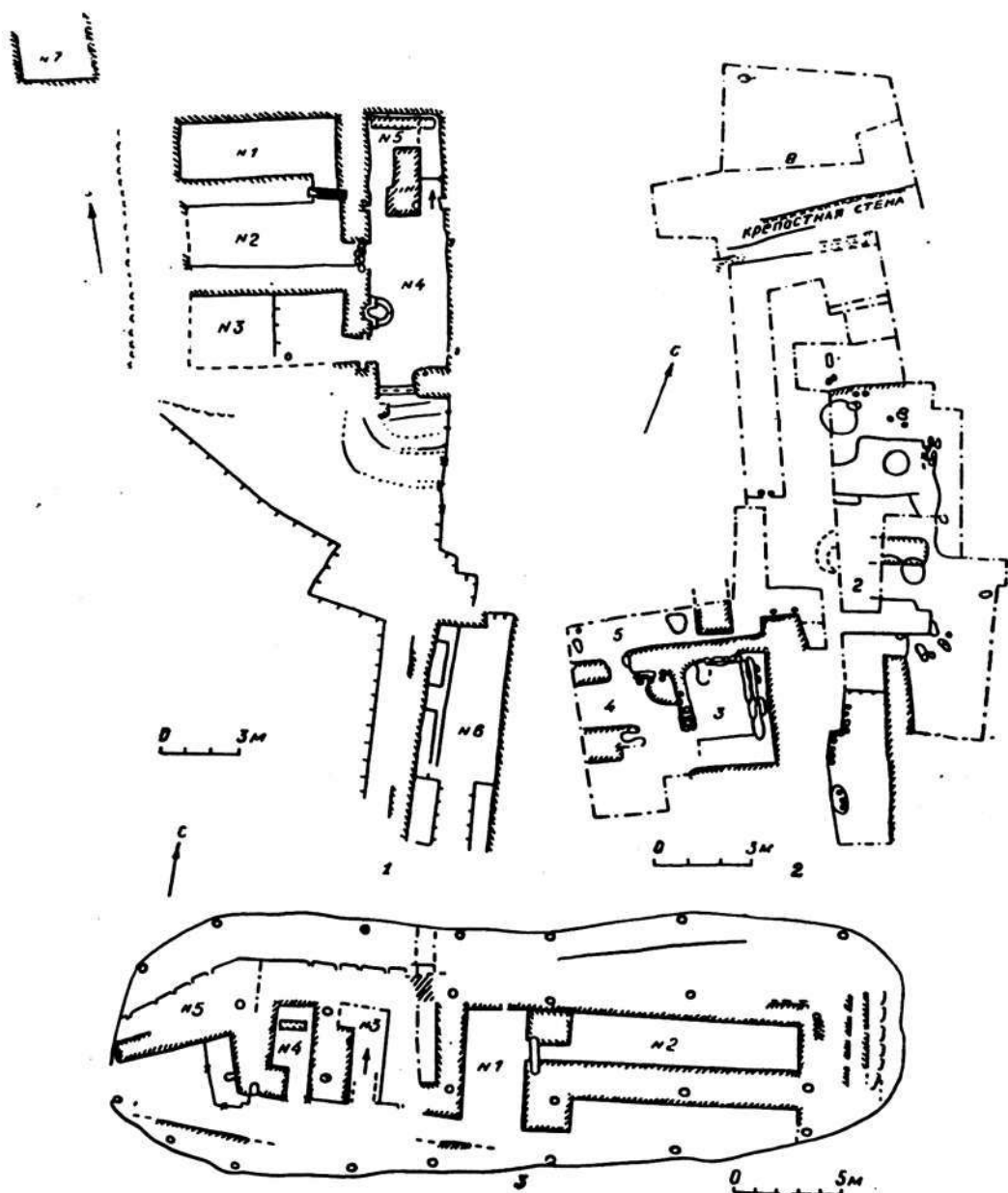
Рис. 3. Планы: 1—Куджара; 2—Қараулато; 3—Қалаи Мирон
