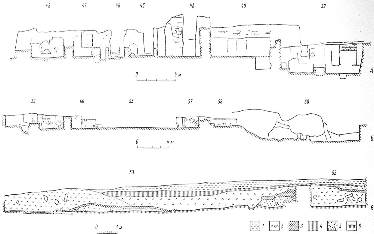
Рис. 4. Разрезы помещений объекта XVI.
