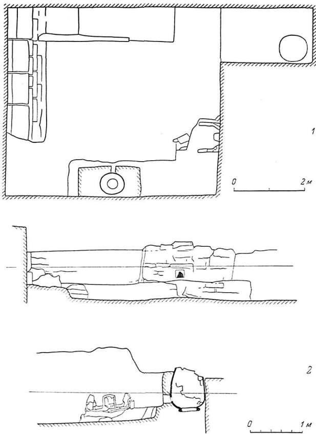
Рис. 17. Педжикент. Объект XVI. Помещение 29. 1 — план; 2 — разрез.
