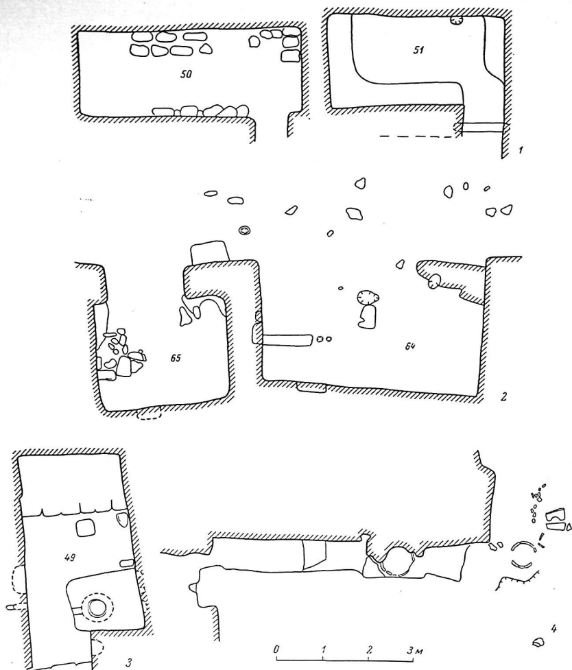
Рис. 18. Пенджикент. Объект XVI. Планы мастерских. — помещения 50, 51; 2 — помещения 65, 64; 3 — помещение 49; 4 — мастерская вдоль южной фасадной стены помещения 62.
