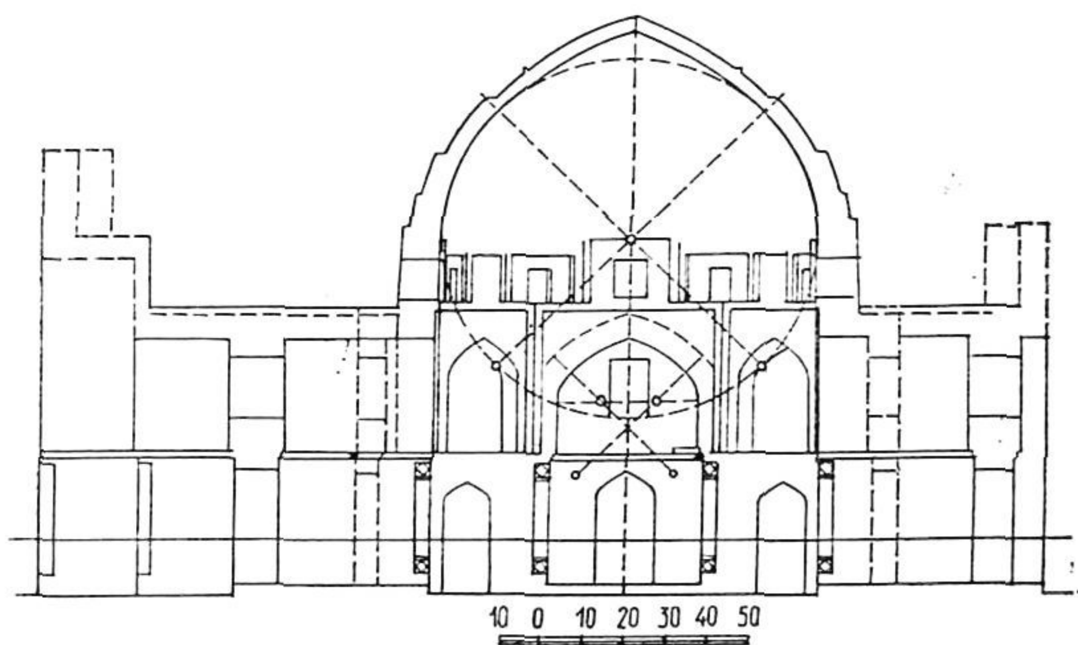
Реконструкция Хонако В. М. Филимонова. Разрез по линии Запад—Восток.
