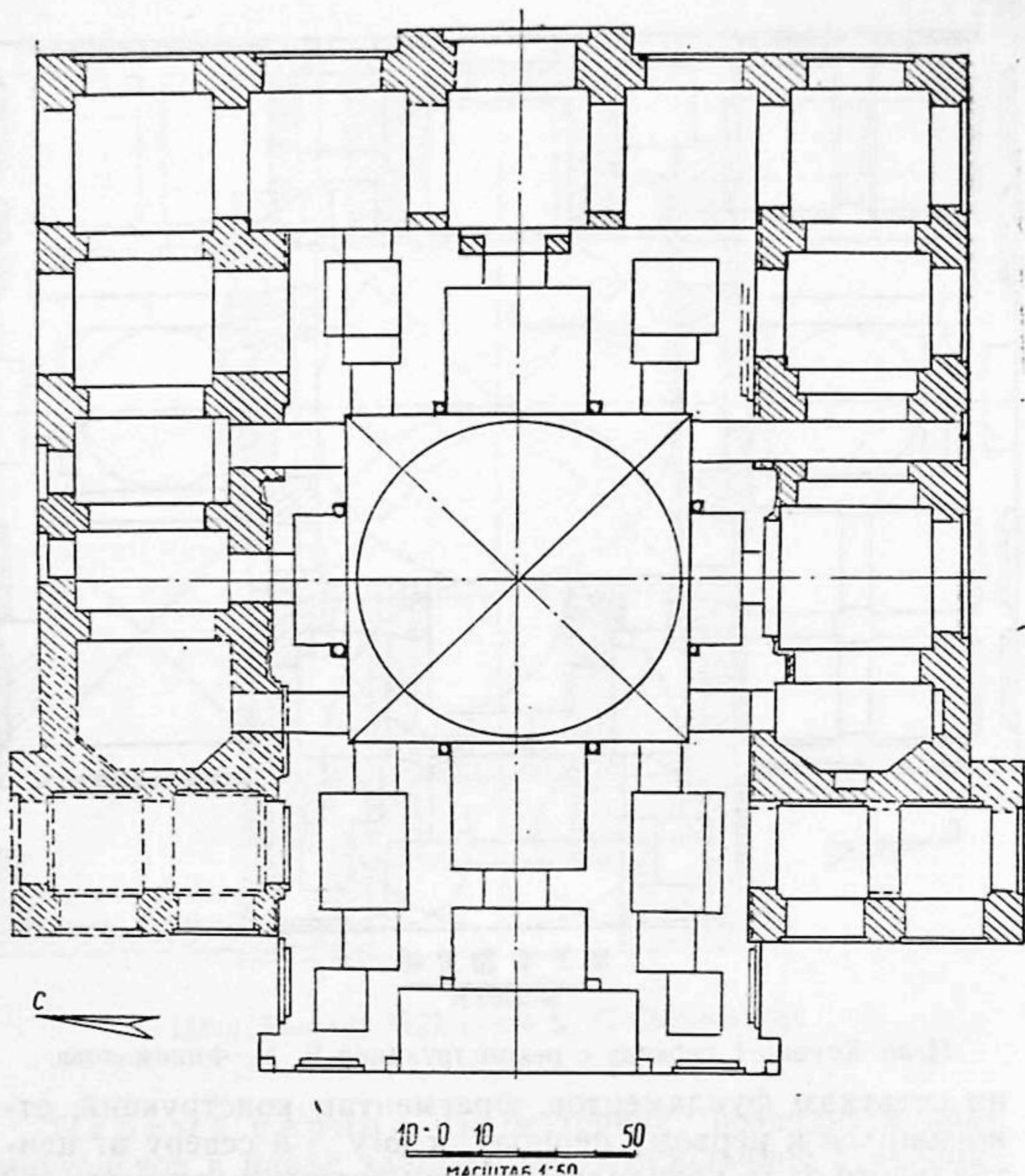
План Хонако II периода с реконструкцией В. М. Филимонова.
