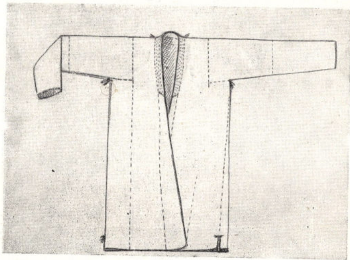
Рис. 56. Раскрой мужского халата.
