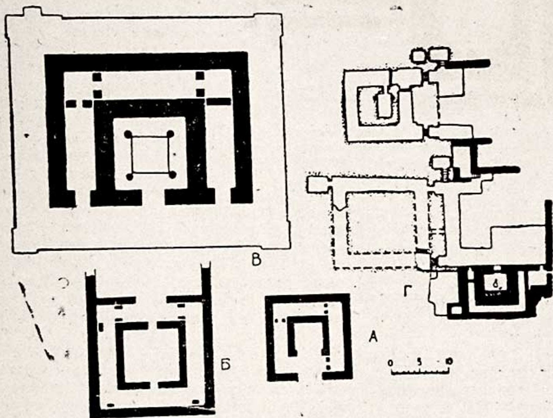
Рис. 4. Композиция. Зал в кулуаре: А — Северный храм на Мансур-депе; Б — Храм на Дальверзине; В — Святилище Канишки в Сурх-Котале; Г — Буддийский монастырь Кара-тепе в Термезе.
