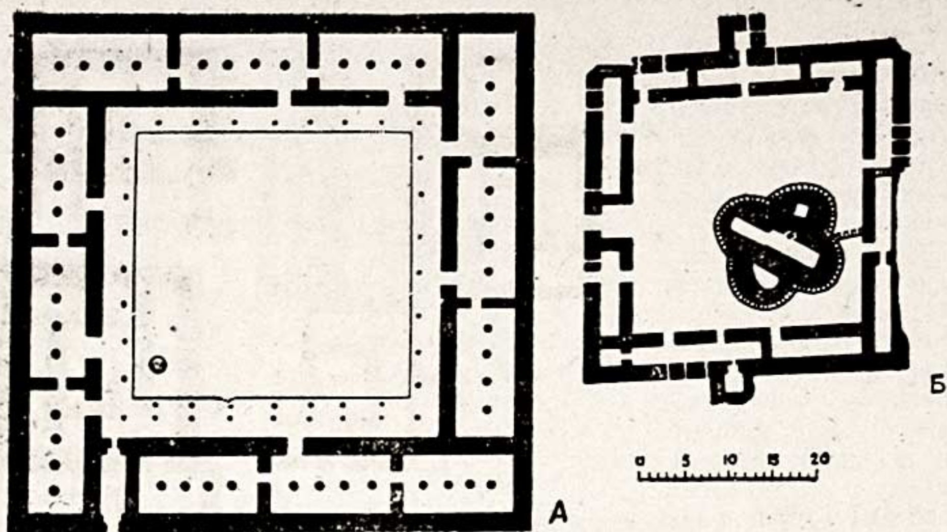
Рис. 7. Композиция. Двор в обводе одного ряда комнат: А — квадратный дом в Старой Нисе; Б — культовый комплекс в Чоб-тобе.
