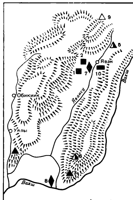
Рис. 12. Памятники Бактрии. Памятники на правобережье р. Вахш (по Б. Я. Ставискому)
