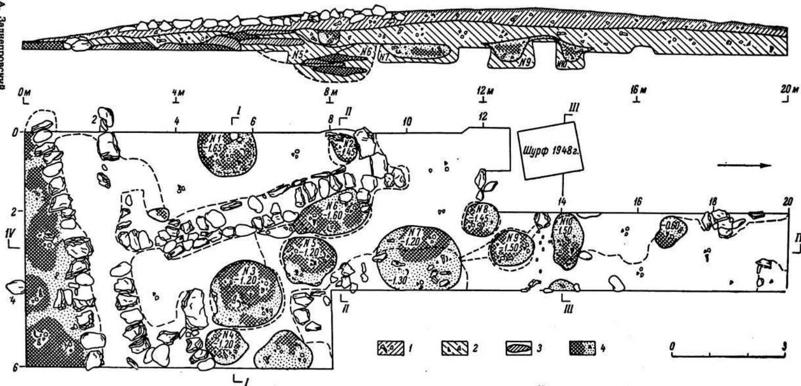
Рис. 40. Даравт-Курганское поселение. План и разрез нижнего горизонта.
